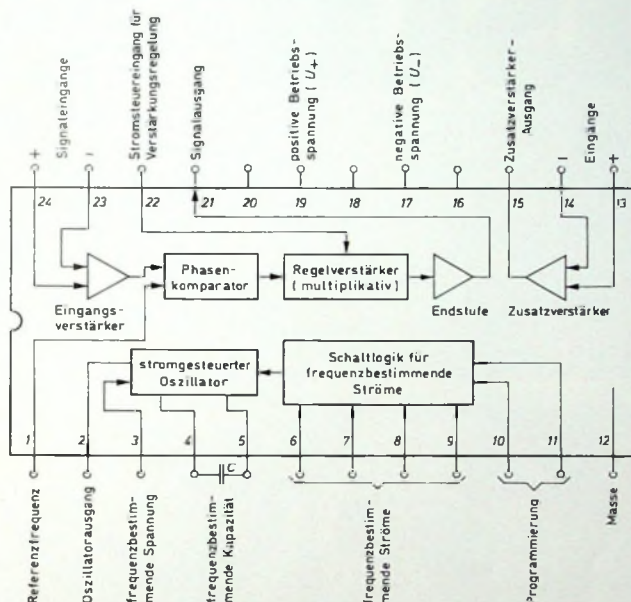
Bild 1. Blockschaltung der integrierten Schaltungen SL 650 und SL 651 mit Anschlußschema
