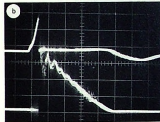
Bild 5 Funkenentladungen einer HKZ nach Bild 2c
