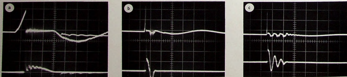
Bild 3. Funkenentladungen einer HKZ nach Bild 2a ( C_n = 1,2 \mu F , U_n = 400 V )
