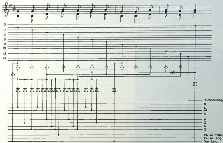
Bild 48 (unten). Printplatte im Maßstab 1:1 zu dem Leitungsplan für das Programmbeispiel im Bild 47
