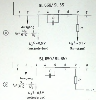
Bild 4. Spannungssteuerung des Oszillators in der SL 650 oder SL 651 über den Anschluß 3; a) der negative Anschluß von R wird an ein konstantes negatives Potential U_R gelegt, b) für U_R wird U_- verwendet
