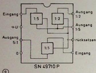
Bild 6. a) Anschlußbelegung der integrierten Schaltung SN 49710 P. b) Prinzip der Erzeugung von 1-Hz-Impulsen aus der Netzfrequenz. c) Schaltung eines 1-Hz-Taktgebers mit der SN 49710 P
