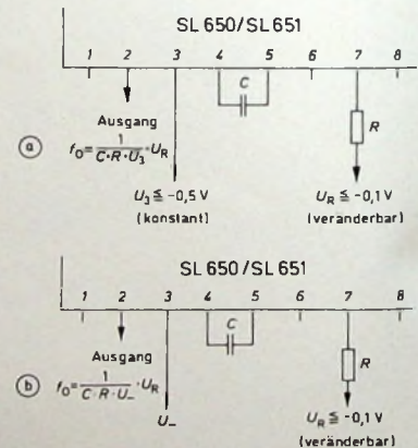
Bild 5. Spannungssteuerung des Oszillators in der SL 650 oder SL 651 mit Hilfe eines Vorwiderstandes vor dem Stromsteuereingang; a) an Anschluß 3 wird ein konstantes negatives Potential gelegt, b) an Anschluß 3 wird U_- gelegt
