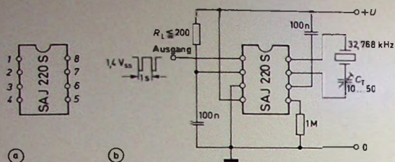
Bild 5. Anschlußbelegung der integrierten Schaltung SAJ 220 S (a) und Schaltung eines quarzstabilen Sekundärtaktgebers mit der SAJ 220 S (b)
