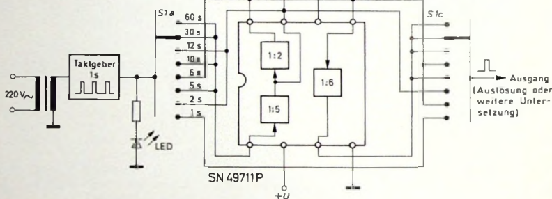
Bild 7. Erweiterung der Schaltung nach Bild 6c durch einen 1:60-Frequenzteiler
