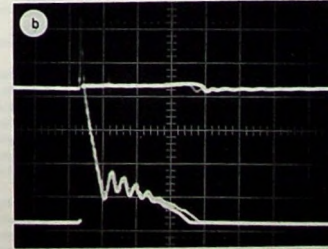
Bild 6 Funkenentladungen einer HKZL nach Bild 2d
