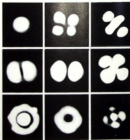
Bild 5. Verschiedene Lichtenergieverteilungen bei wachsendem Durchmesser der Glasfaser
