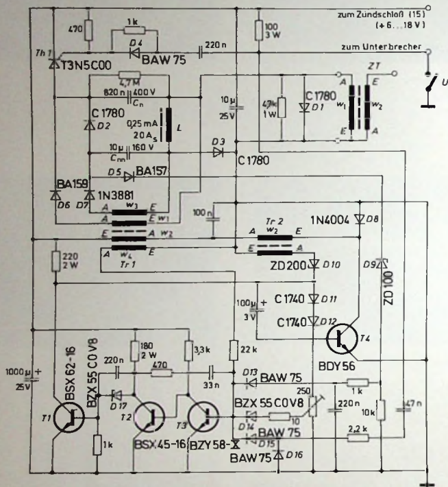
Bild 7. Beispiel einer HKZ für 12-V-Betrieb mit einer Funkenstandzeit von etwa 0,3 ms
