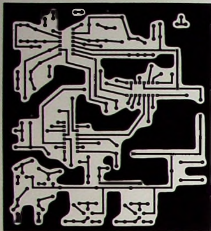
Bild 3. Printplatte des SQ-Logic-Decoders im Maßstab 1:2 (Leiterbahenseite)
