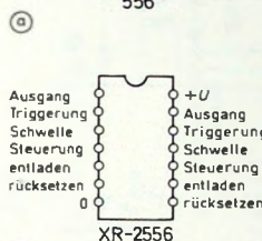
Bild 3. Anschlußbelegung der integrierten Schaltungen 556 (a) und XR-2556 (b) sowie Schaltung eines Doppel-Zeitgebers mit der XR-2556 (c)
