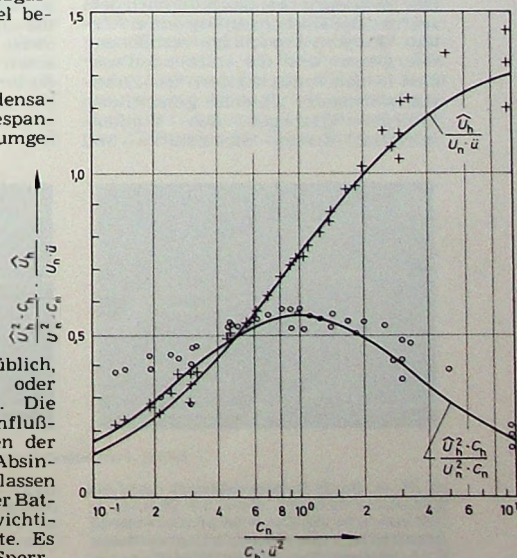
Bild 1. Erreichbare Hochspannung \hat{U}_h und übertragene Energie für HKZ in Abhängigkeit von der Kapazität des Speicherkondensators
