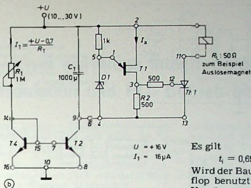
Bild 2. a) Schaltung des Thyristor-Transistor-Arrays CA 3097 E, b) Zeitrasterfahrschaltung der CA 3097 E (Dimensionierung für 8,3 min)
