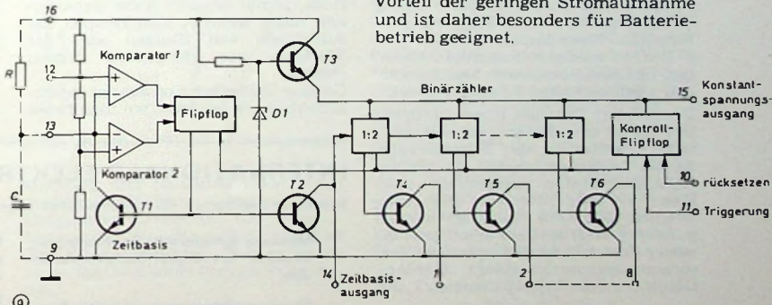
Bild 4. Prinzipschaltung und Anschlußbelegung der integrierten Schaltung XR-2240 (a) und Anwendungsbeispiele mit der XR-2240 (b, c)
