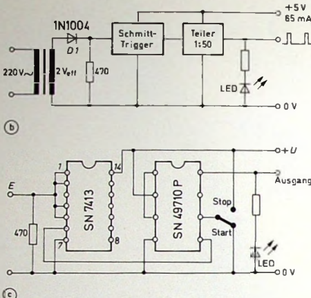
Bild 6. a) Anschlußbelegung der integrierten Schaltung SN 49710 P. b) Prinzip der Erzeugung von 1-Hz-Impulsen aus der Netzfrequenz. c) Schaltung eines 1-Hz-Taktgebers mit der SN 49710 P
