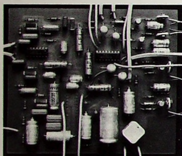
Bild 5. Bestückte Printplatte (Bestückungsseite)
