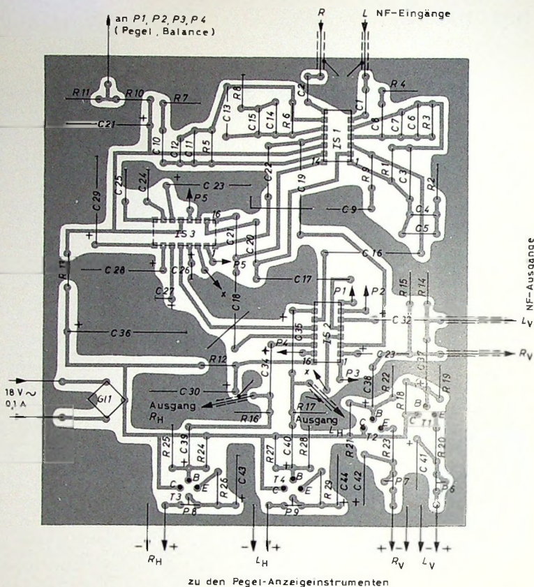
Bild 3. Printplatte des SQ-Logic-Decoders im Maßstab 1:2 (Leiterbahenseite)
